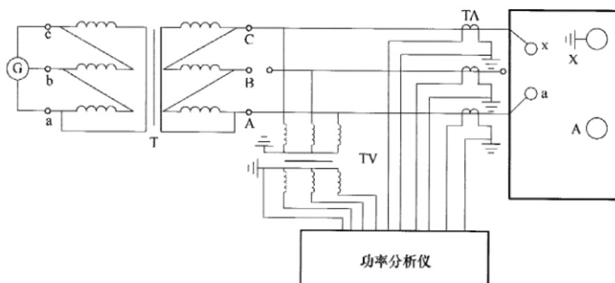
图5 三相变压器空载试验接线示意图（油浸式电力变压器）
