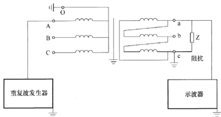
图20 暂态电压传输特性试验接线示意图
