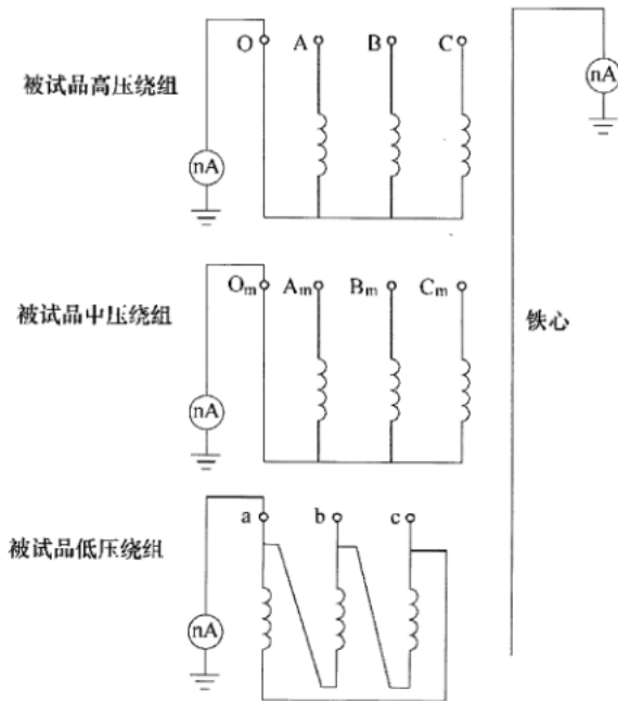
图23 油流静电试验接线示意图
