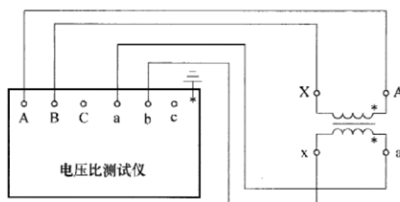
图25 单相变压器电压比测量接线示意图（干式电力变压器）
