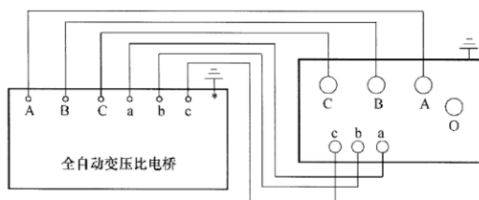
图2 三相变压器电压比测量接线示意图（油浸式电力变压器）
