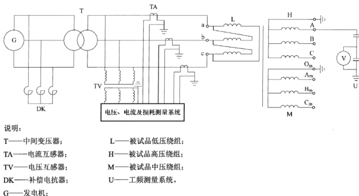
图8 感应耐电压试验典型接线示意图（油浸式电力变压器）
