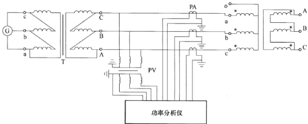
图29 单相变压器空载试验接线示意图（干式电力变压器）
