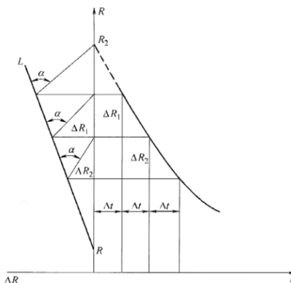
图39 确定切断电源瞬间热电阻温度的方法
