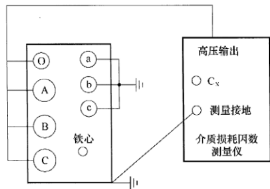
图13 绕组对地电容测量接线示意图（“反接”法）
