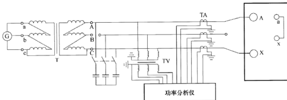
图3 三相变压器负载试验接线示意图（油浸式电力变压器）
