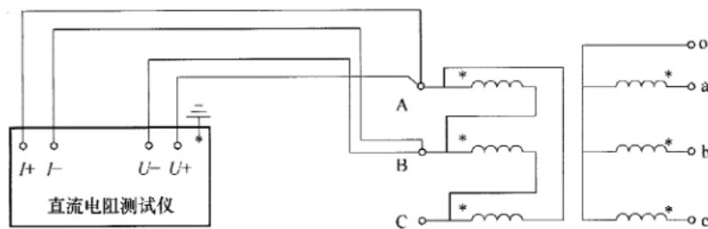
图24 绕组电阻测量试验接线示意图
