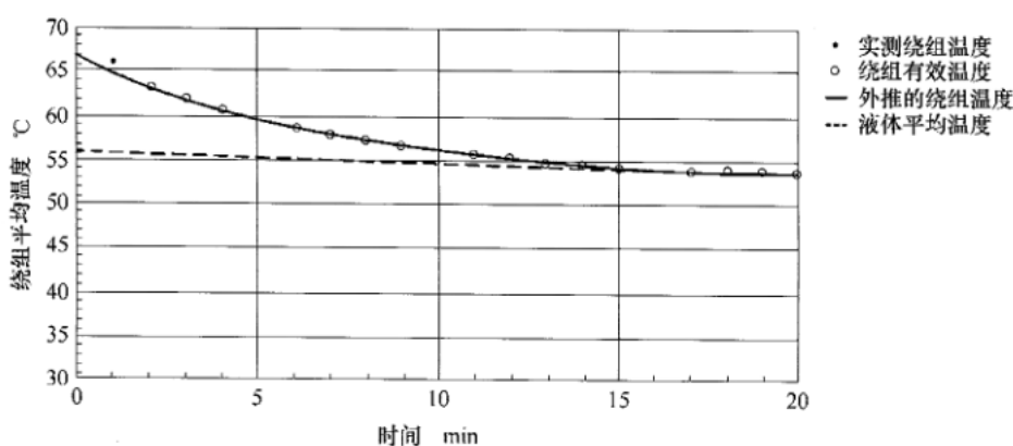
图14 计算机程序外推冷却曲线
