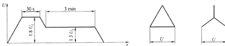
图35 局部放电例行试验的施加电压方式
