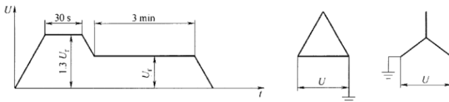
图36 局部放电特殊试验的施加电压方式
