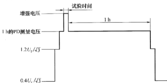
图10 带有局部放电测量的感应耐电压试验施加电压的时间顺序
