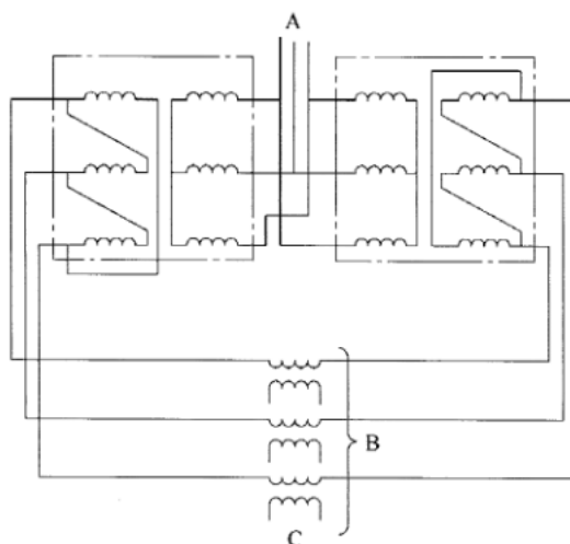
图37 单相相互负载法接线示意图
