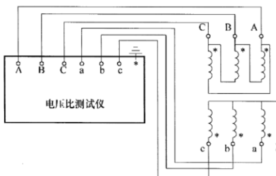
图26 三相变压器电压比测量接线示意图（干式电力变压器）
