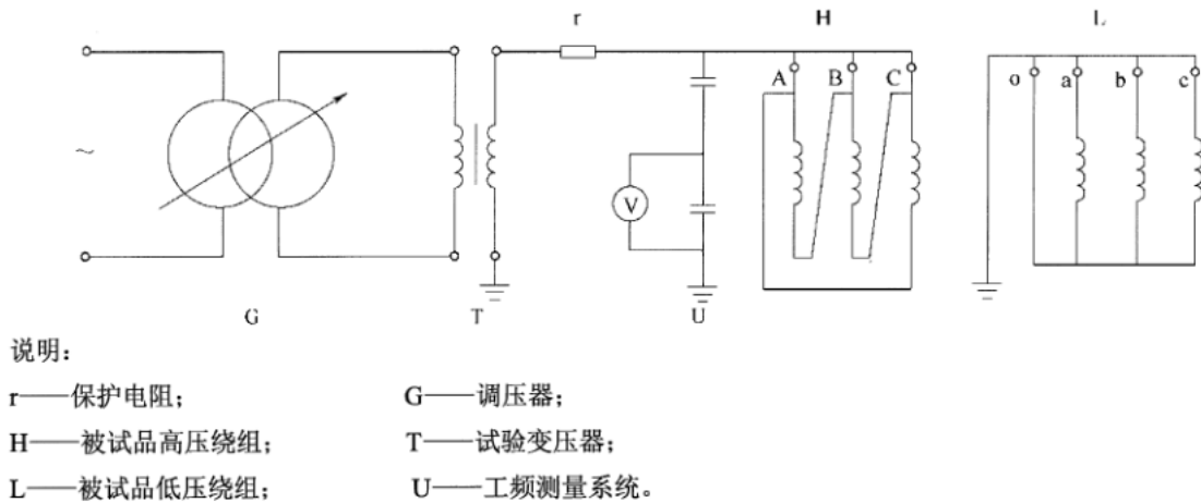
图31 外施耐电压试验接线示意图（干式电力变压器）
