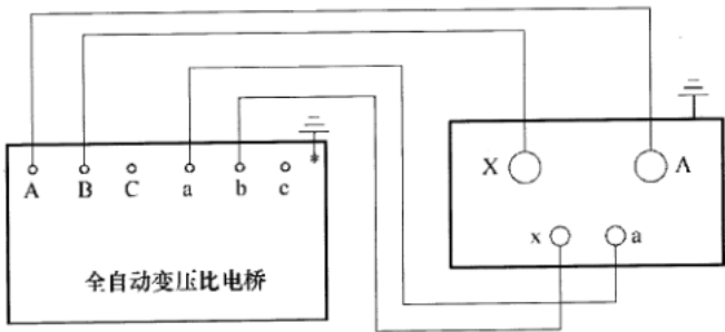
图1 单相变压器电压比测量接线示意图（油浸式电力变压器）
